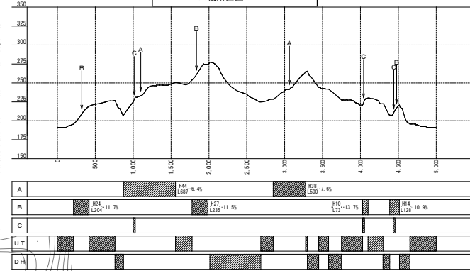
十日町市吉田クロスカントリー競技場 5km-Aコース縦断面図
