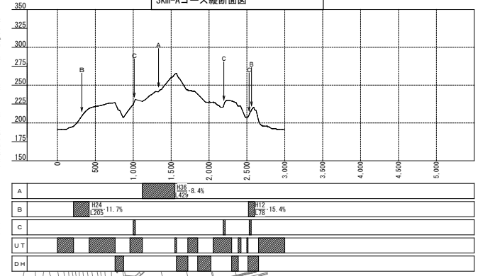
十日町市吉田クロスカントリー競技場 3km-Aコース縦断面図
